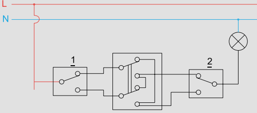
Bağlantı Şeması Wiring Diagram
