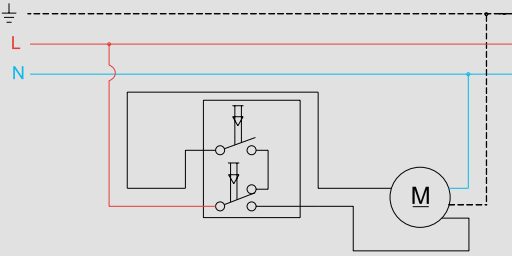
Bağlantı Şeması Wiring Diagram
