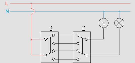
Bağlantı Şeması Wiring Diagram
