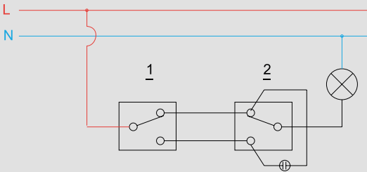
Bağlantı Şeması Wiring Diagram
