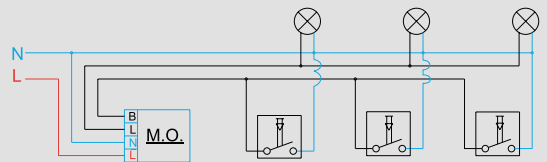
Bağlantı Şeması Wiring Diagram
