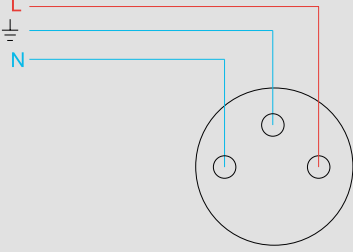
Bağlantı Şeması Wiring Diagram
