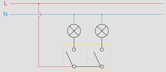
Bağlantı Şeması Wiring Diagram
