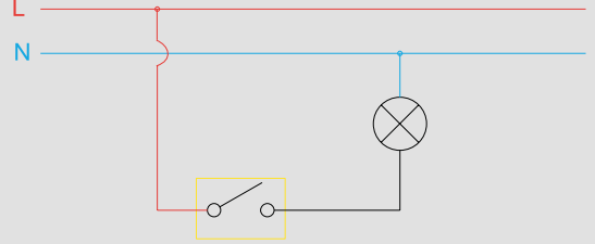
Bağlantı Şeması Wiring Diagram
