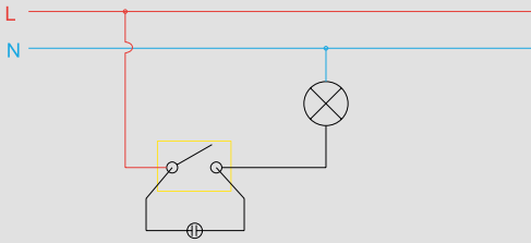
Bağlantı Şeması Wiring Diagram
