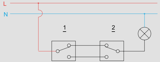
Bağlantı Şeması Wiring Diagram
