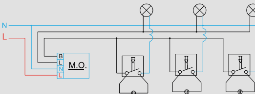
Bağlantı Şeması Wiring Diagram
